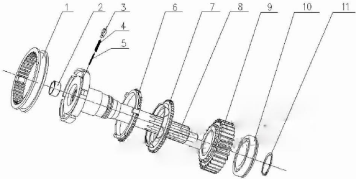
输入轴及齿轮总成
