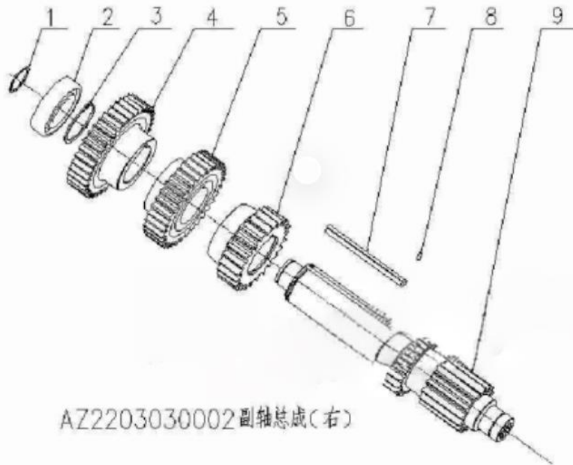
副轴总成（右）
