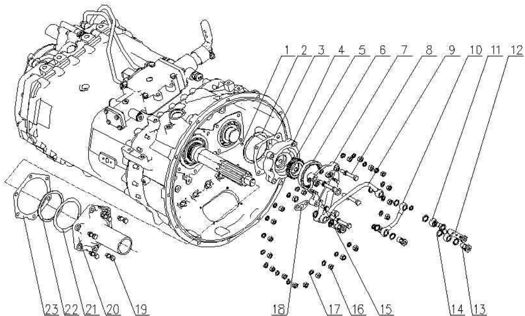
变速器总成（六）
