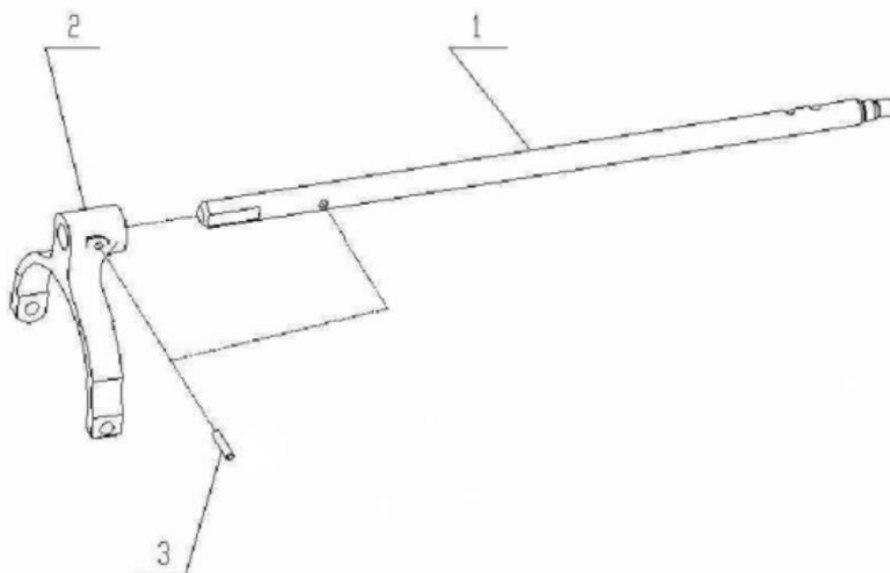
插分档拨叉轴总成
