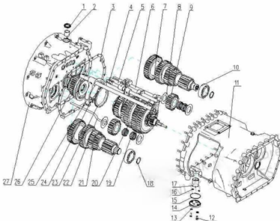
变速器总成（四）
