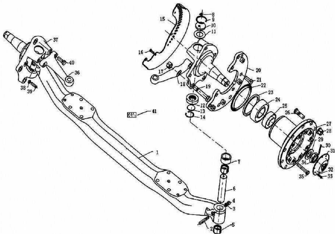
前轴总成 (HR9, ABS, 分体式转向节, 带防护罩)
