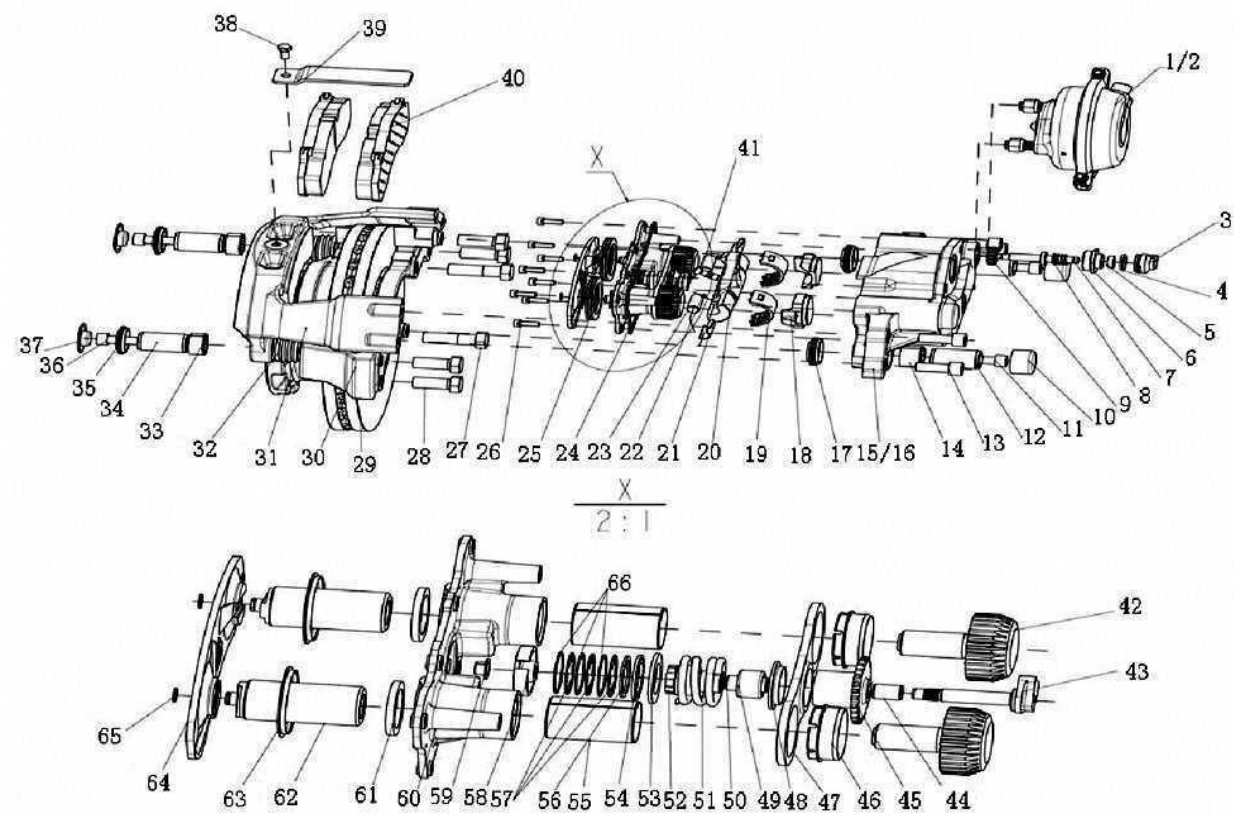
第二代应用型盘式制动器
