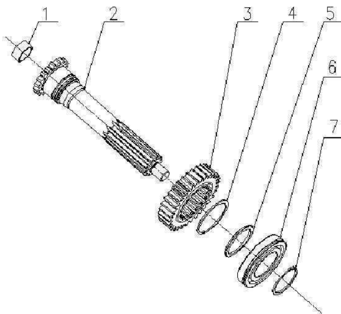
输入轴及一轴齿轮总成
