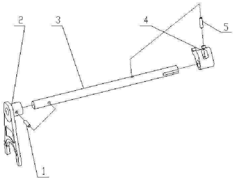
倒档拨叉轴总成
