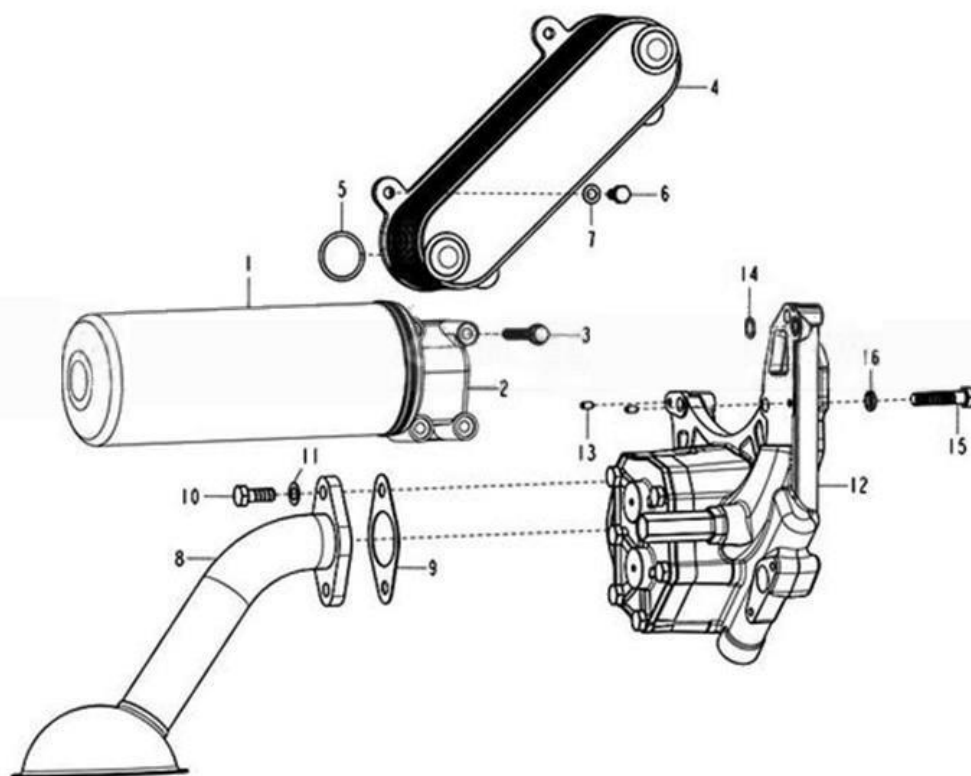
机油泵和滤清器
