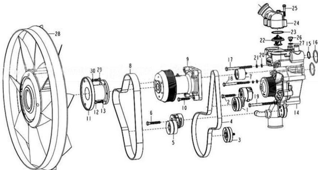
水泵和冷却系统
