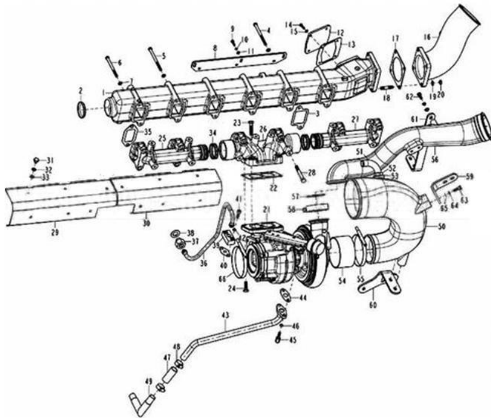
进排气系统
