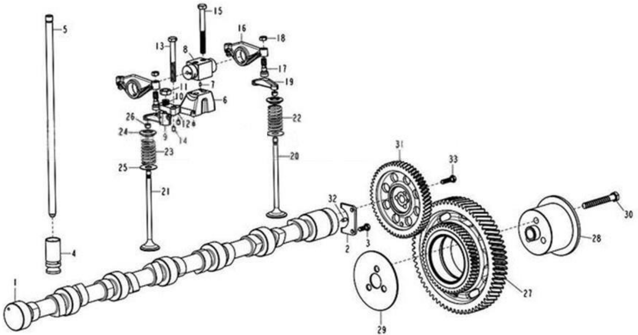
配气机构
