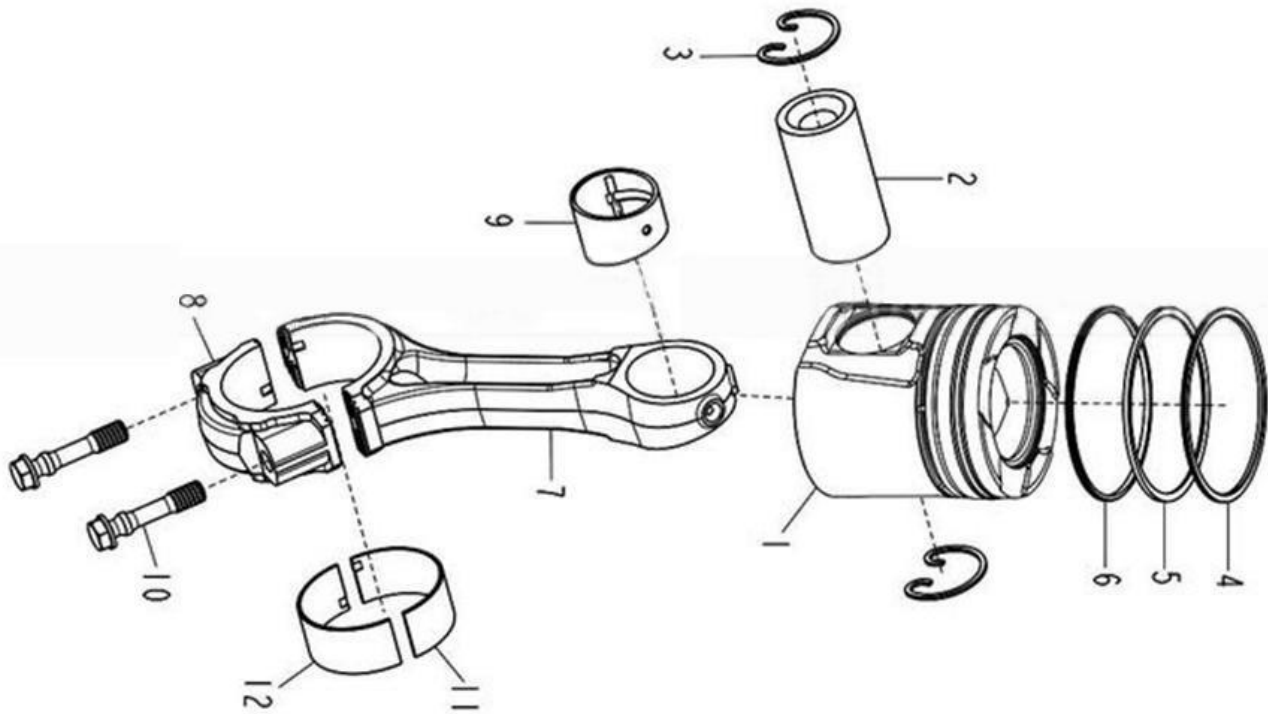
活塞和连杆
