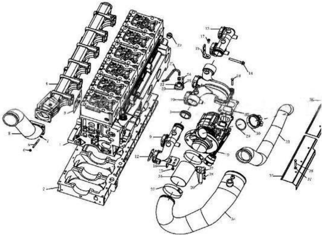
进排气部分（四气门中置）
